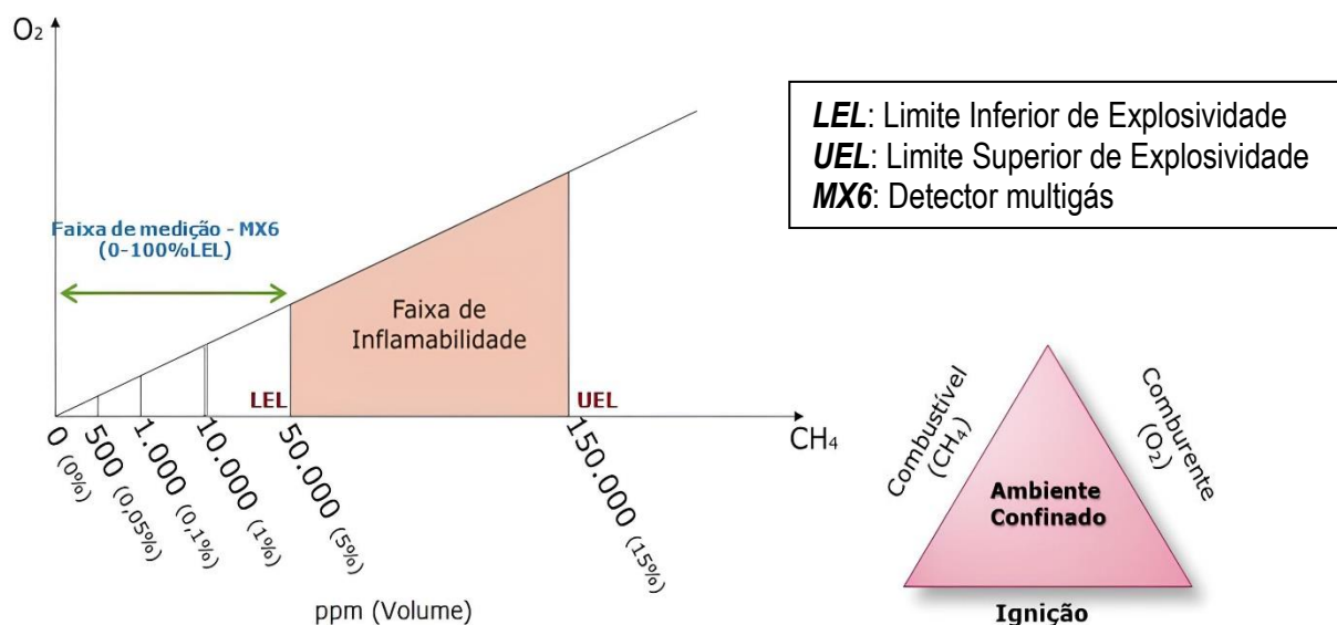
Figura 2. Esquema da faixa de inflamabilidade do metano e sua combustão
