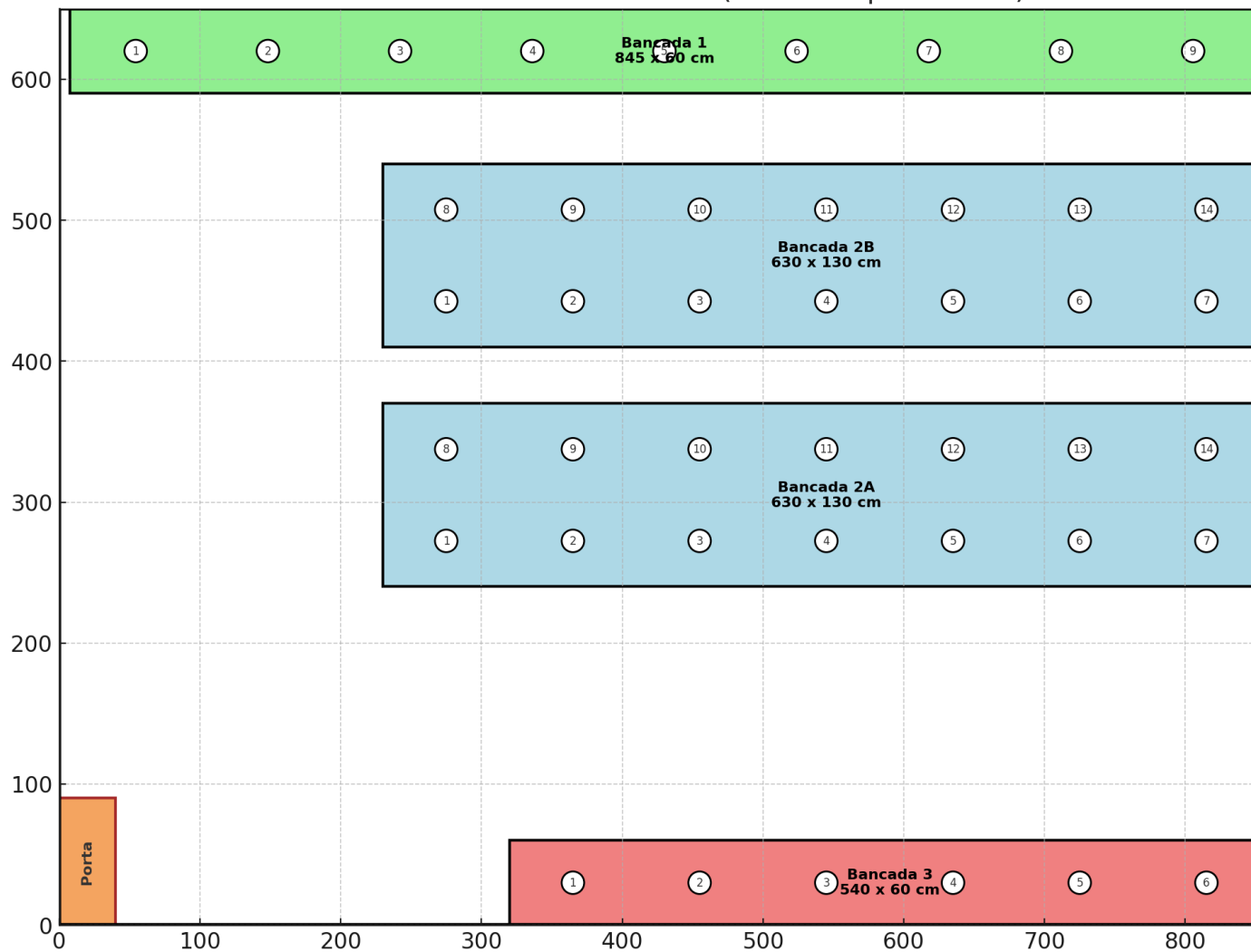
Planta Baixa - Laboratório 1 (com computadores)
