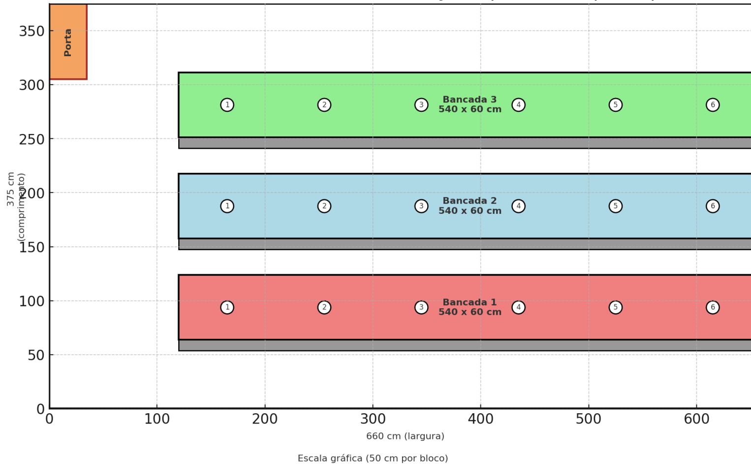
Planta Baixa - Laboratório 3 (18 estações, porta no topo esquerdo)
