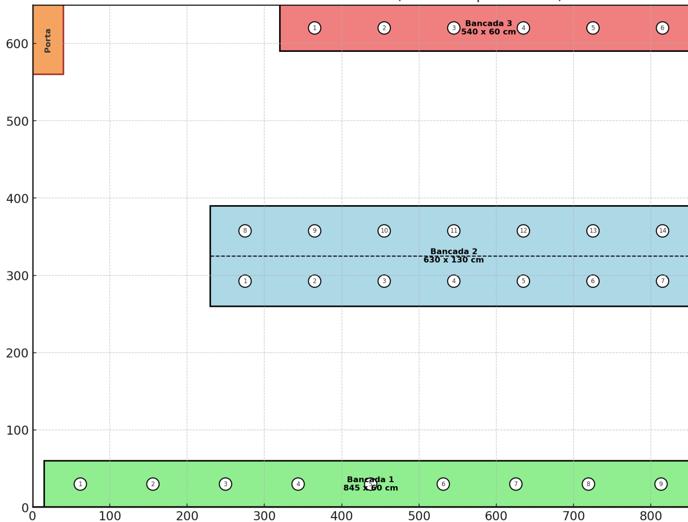
Planta Baixa - Laboratório 2 (com computadores)
